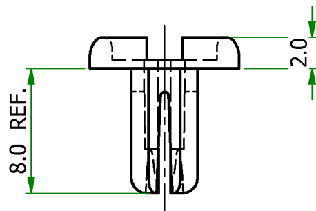
GROMMET
